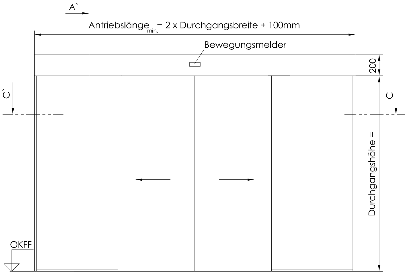
Ansicht X
