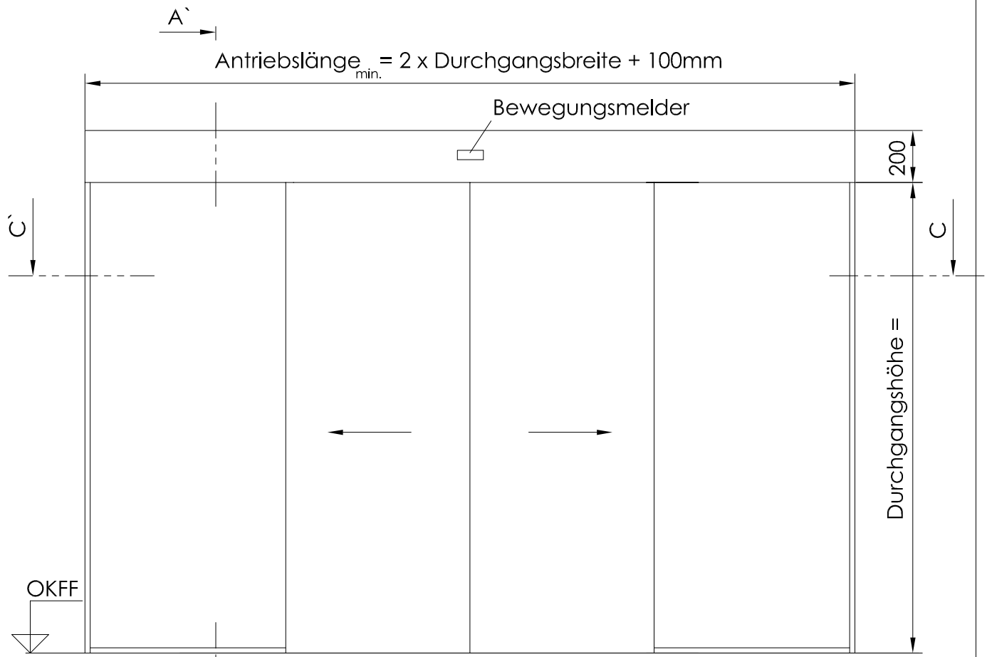
Ansicht X
